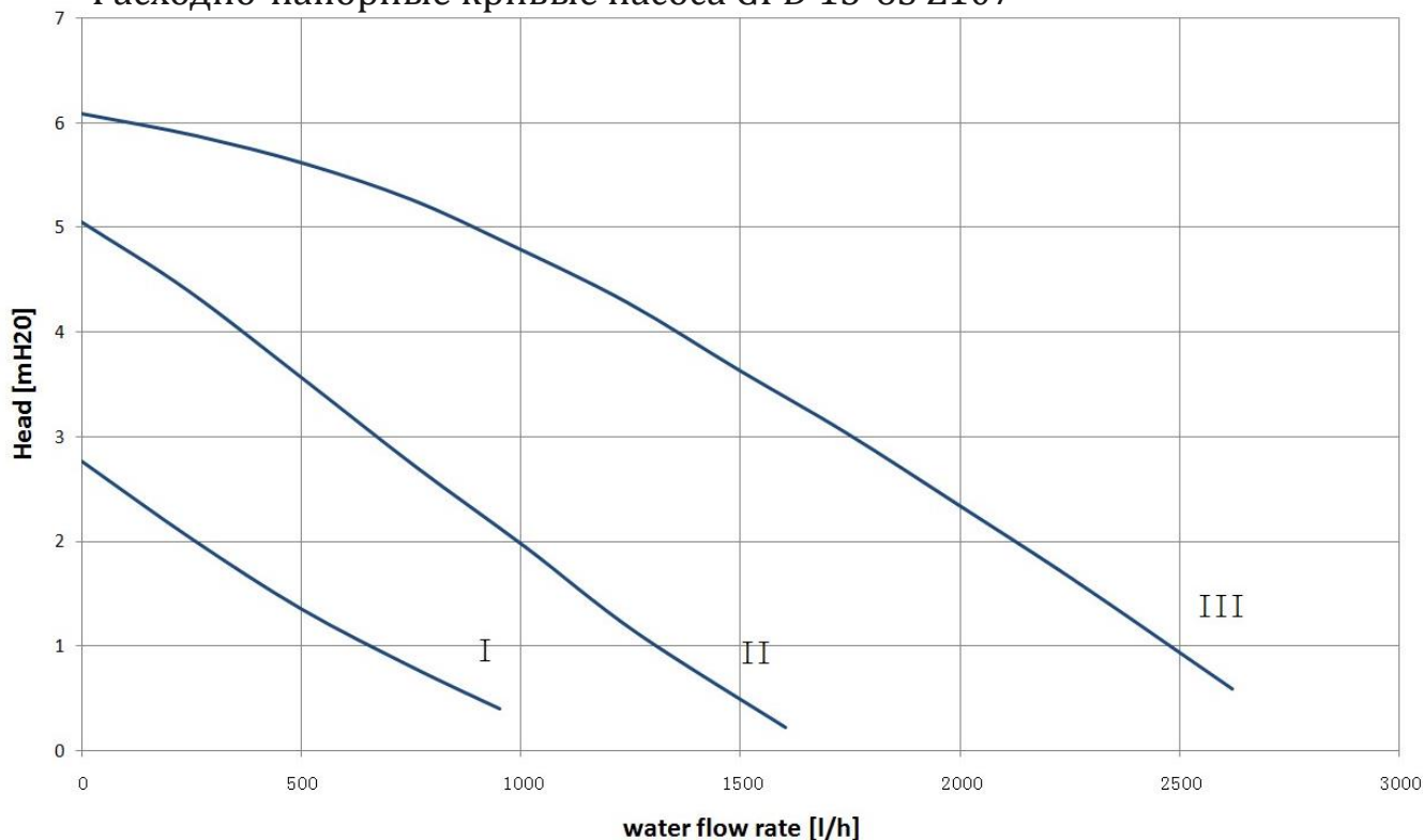
Расходно-напорные кривые насоса GPD 15-6S Z107
