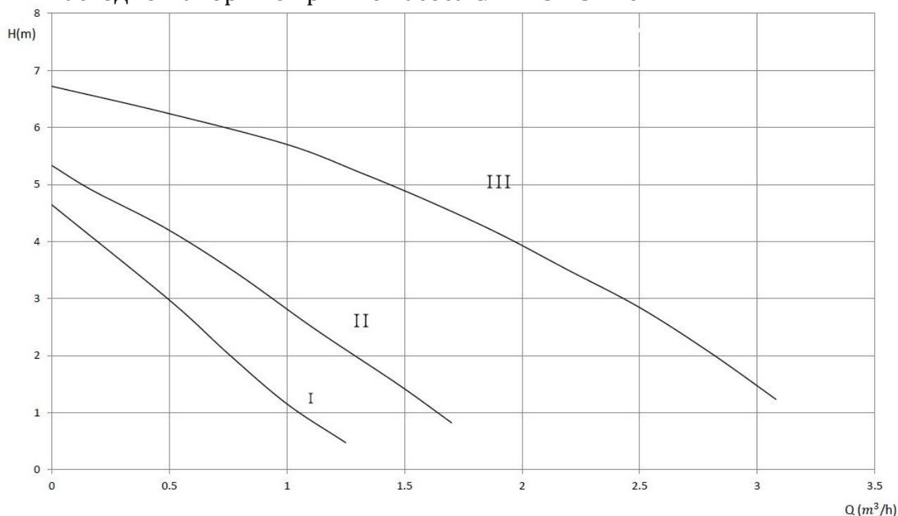
Расходно-напорные кривые насоса GPD 15-7S Z107
